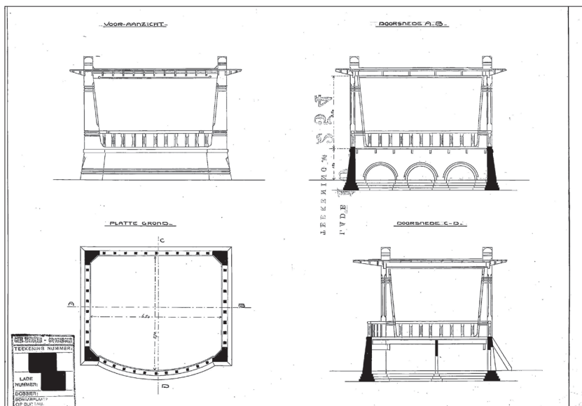
Afb. 12. Ontwerp van een muziektent in het Noorderplantsoen van J.A. Mulock Houwer, 1905. Dienst Ruimtelijke ordening/Economische zaken, werktekeningen 1860-1990, collectie RHC Groninger Archiven (1615-480).
